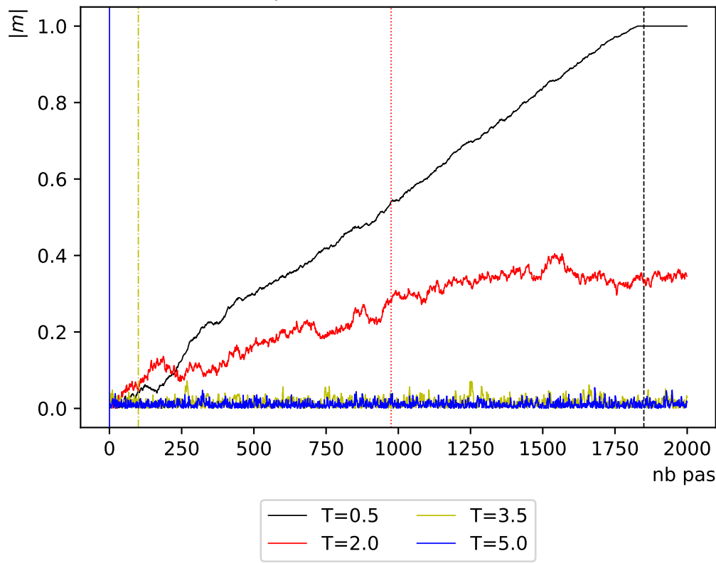
Evolution selon critère Estimation par intervalle,Condition Initiale aléatoire de taille L=128
